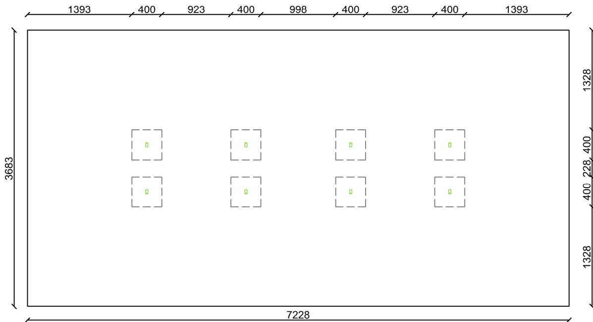
PLANIMETRIA DELLE BUCHE (HOLES PLANIMETRY)
